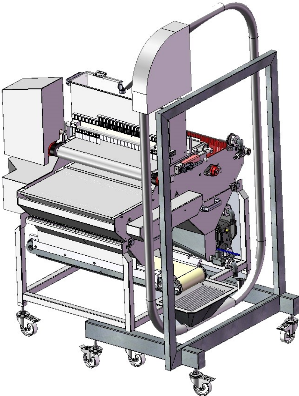
Sesamstreuer mit Saatenrückführung
